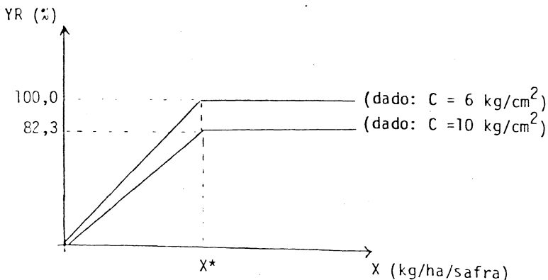
FIG. 1. Resposta relativa dos cultivos (YR) à aplicação de fertilizantes (X) sob níveis diferenciados de compactação na base da camada arada (C).
